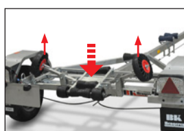
Selvjusterende vugge
